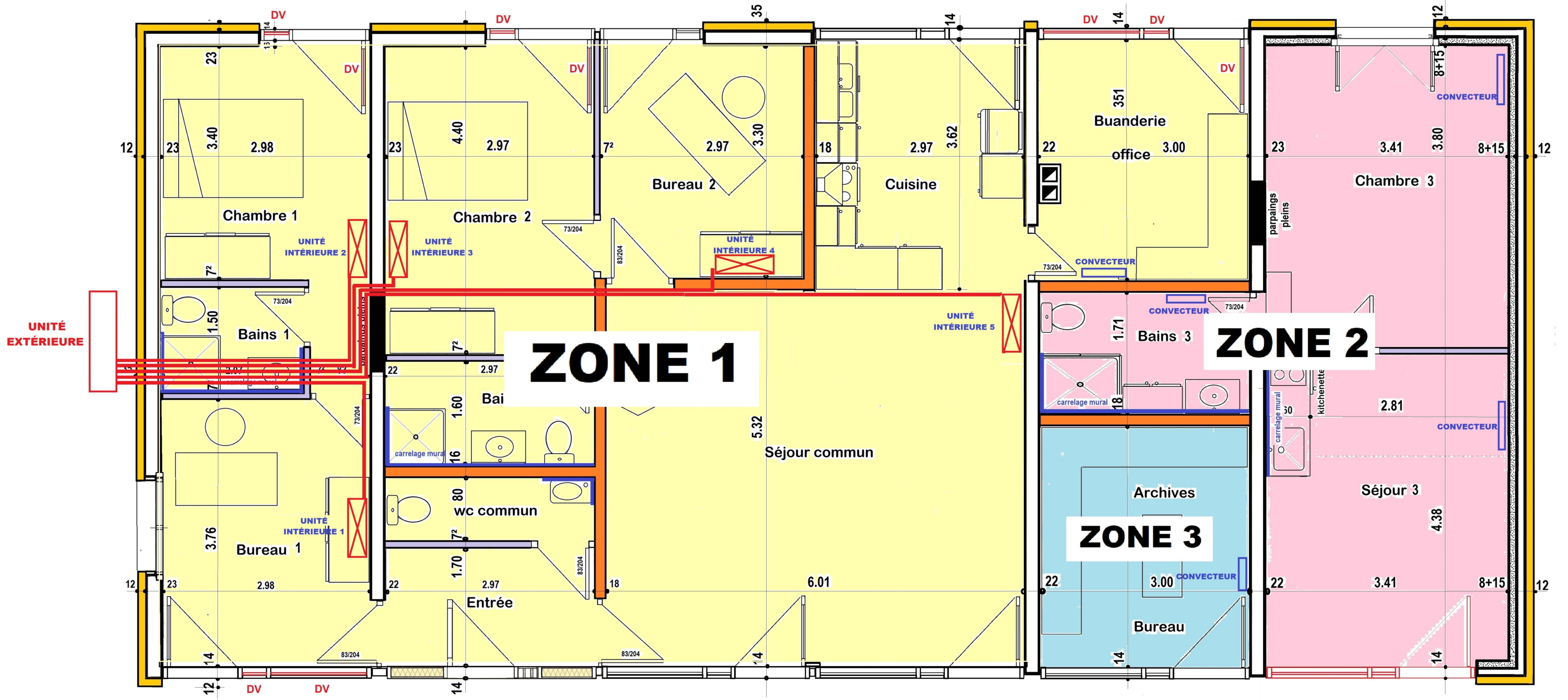
06A PLAN ZONAGE CHAUFFAGE éch. : 1/50ème
